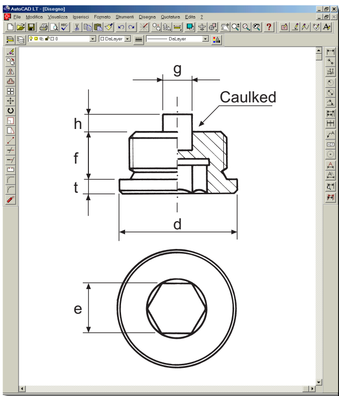
NORMA DIN 908 type
